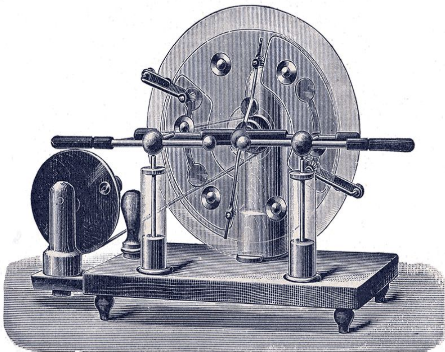
Fig. 304 Töpler'sche Elektrifiziermaschine
