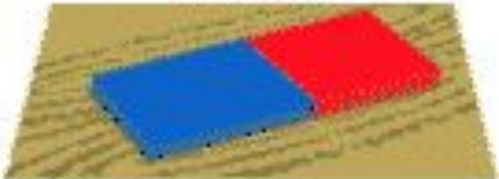
Расположение опилок в поле полосового магнита
