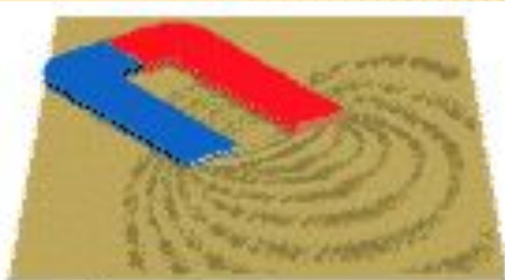
Расположение опилок в поле подковообразного магнита
