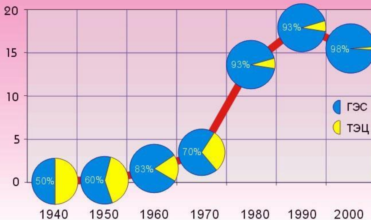
Производство электроэнергии гидро и теплоэлектростанциями в Таджикистане (млрд. кВт. ч.)
