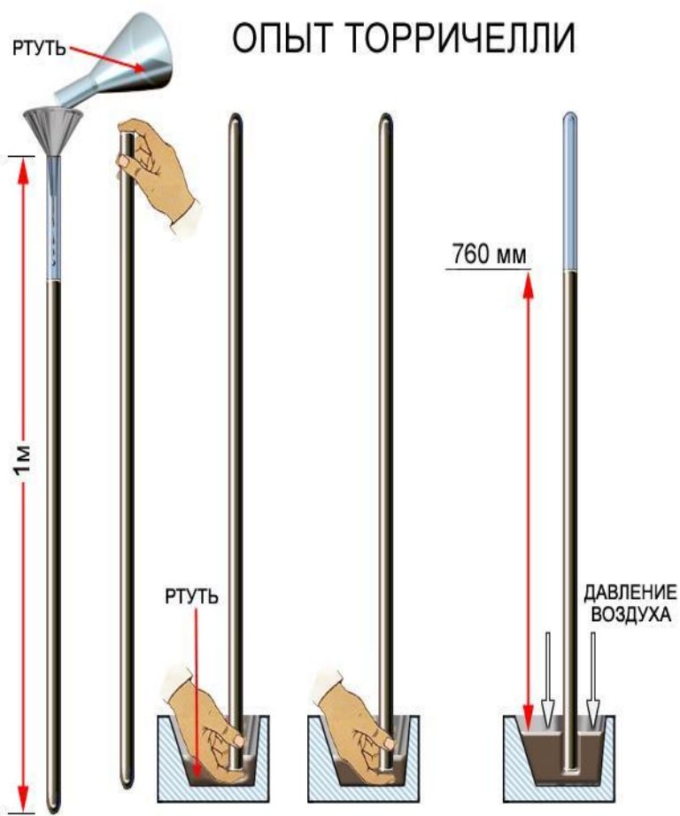
СХЕМАТИЧЕСКОЕ УСТРОЙСТВО РТУТНОГО БАРОМЕТРА
