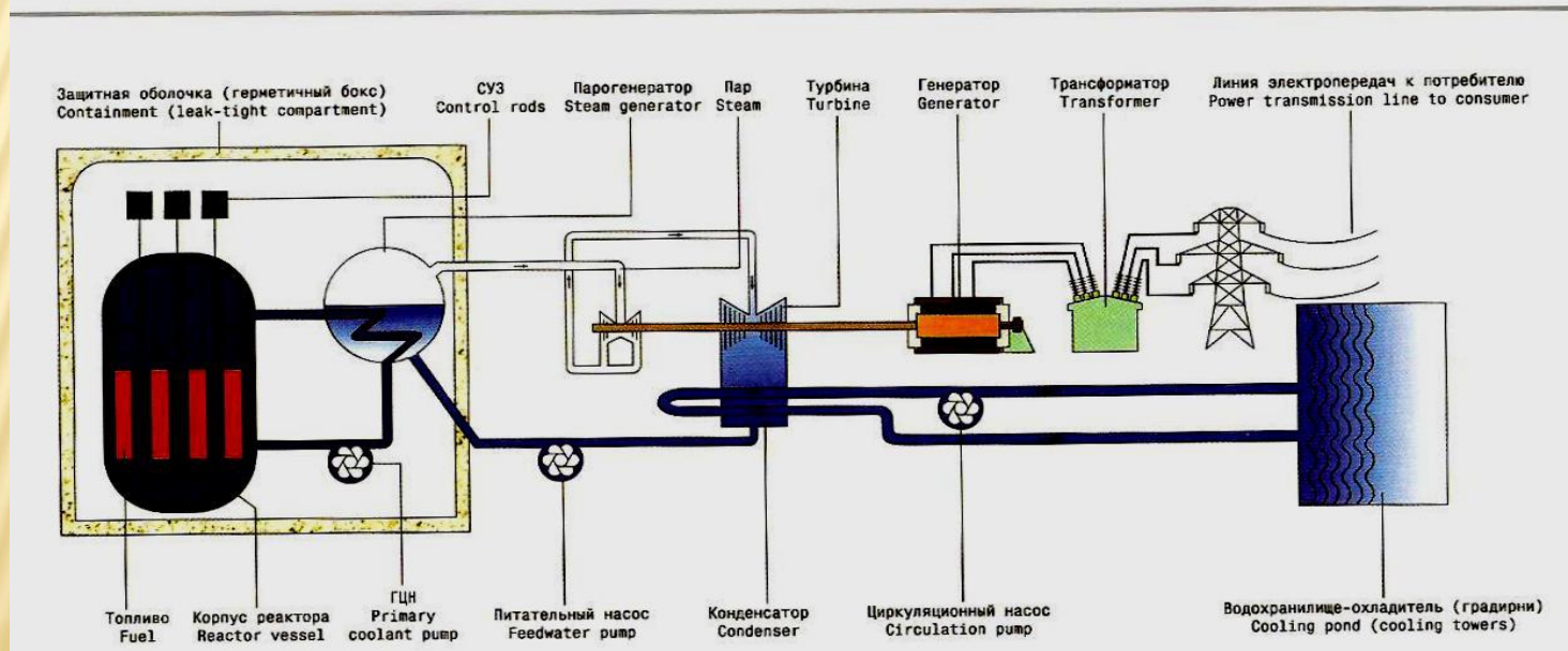
Технологическая схема энергоблоков / Power Unit Flow Diagram
