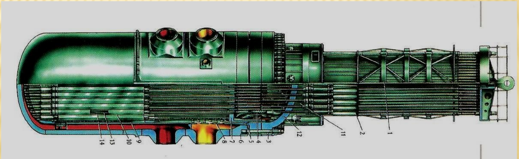
ВВЭР-1000
