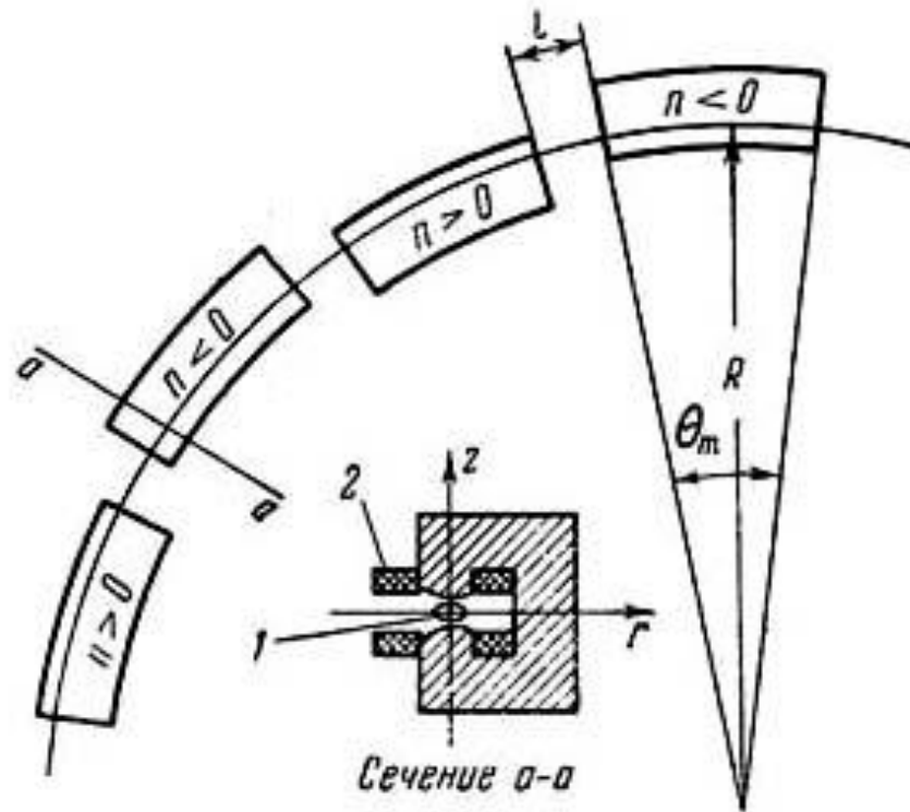
Схема сильнофокусирующего синхрофазотрона: \theta_m — угловой размер магнитного блока; l — длина промежутка, свободного от поля; 1 — поперечное сечение вакуумной камеры; 2 — обмотки магнита (изображение: «Наука и жизнь»)
