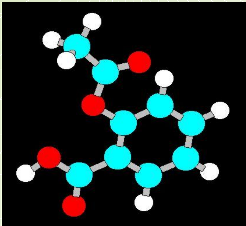
Молекула аспирина
