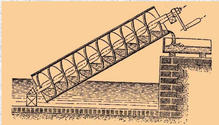
Архимедов винт
