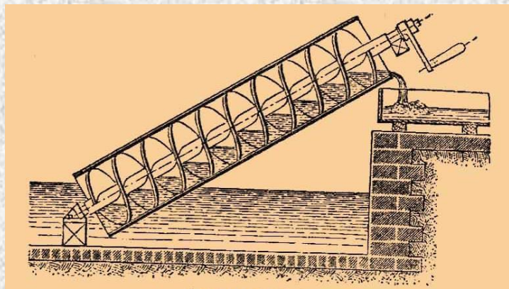
Архимедов винт
