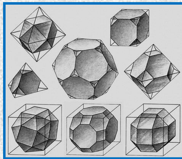
ПОЛУПРАВИЛЬНЫЕ МНОГОГРАННИКИ
