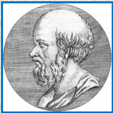
Эратосфен
