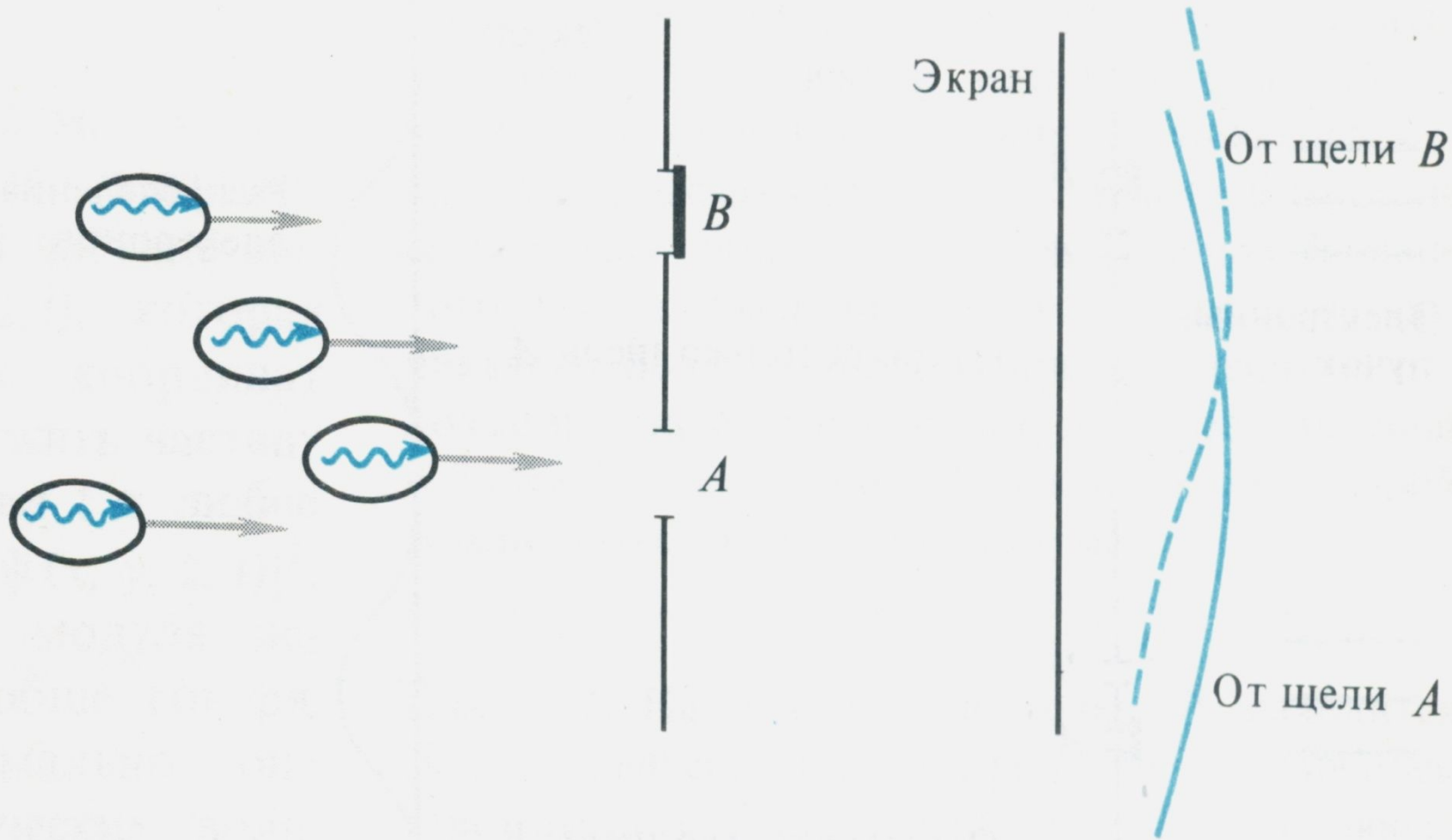
Рис. 7. Распределение интенсивности, обусловленное фотонами, прошедшими через щель A (либо через щель B)
