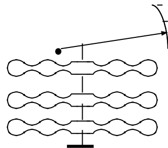
Рис. 4.2.2. Сильфон.
