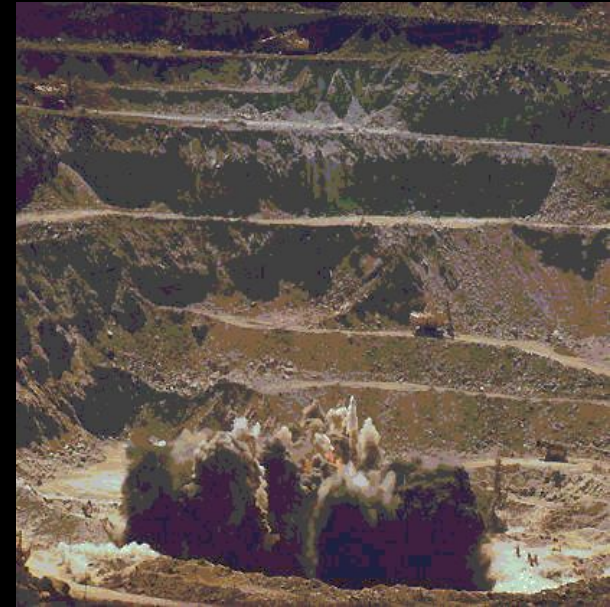
жарылыстар
