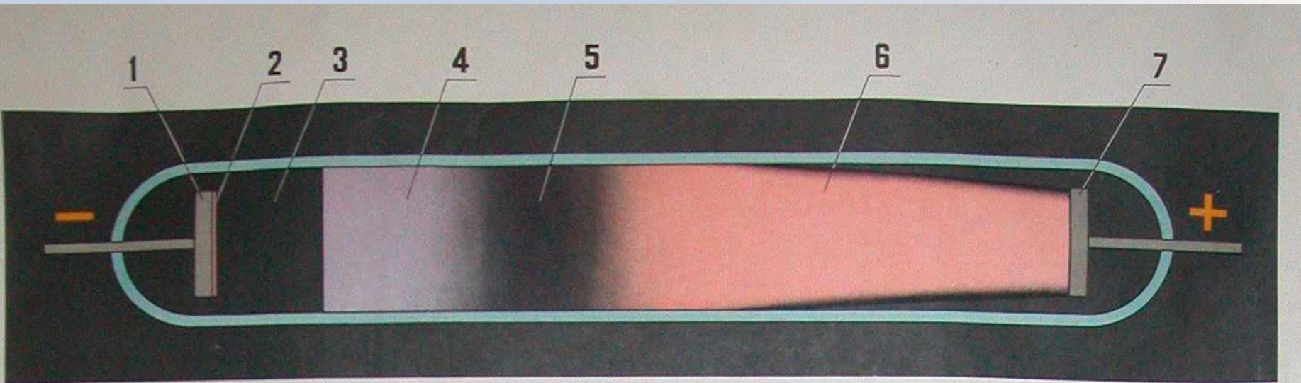
КАТОДНАЯ ТРУБКА
