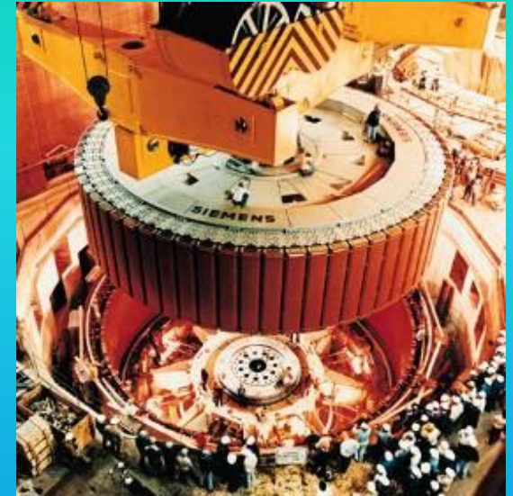
Генератор
