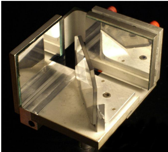
Блок зеркал интерферометра
