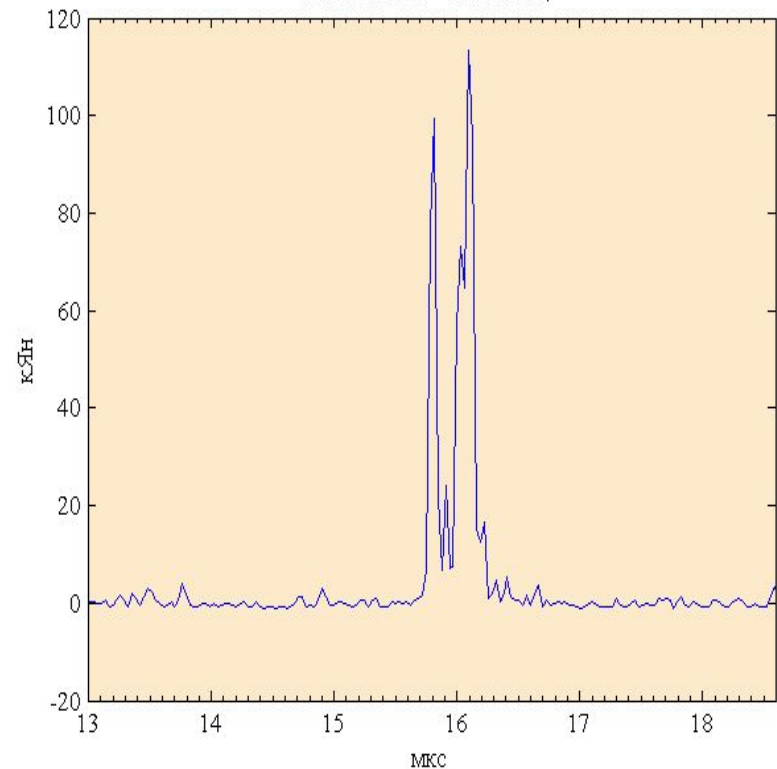
PSR 0531+21 2200 МГц
