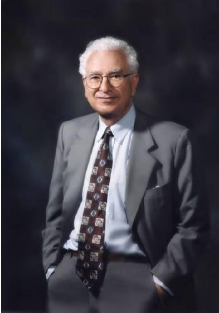
М. Гелл-Манн
