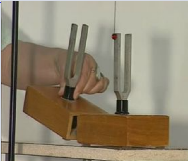
Резонанс звука
