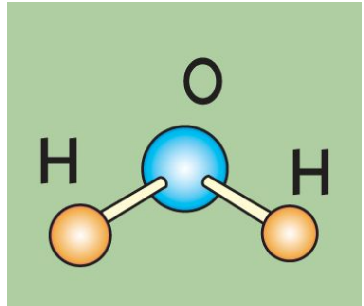
Молекула воды
