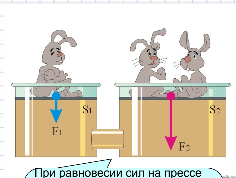
Гидравлический пресс
