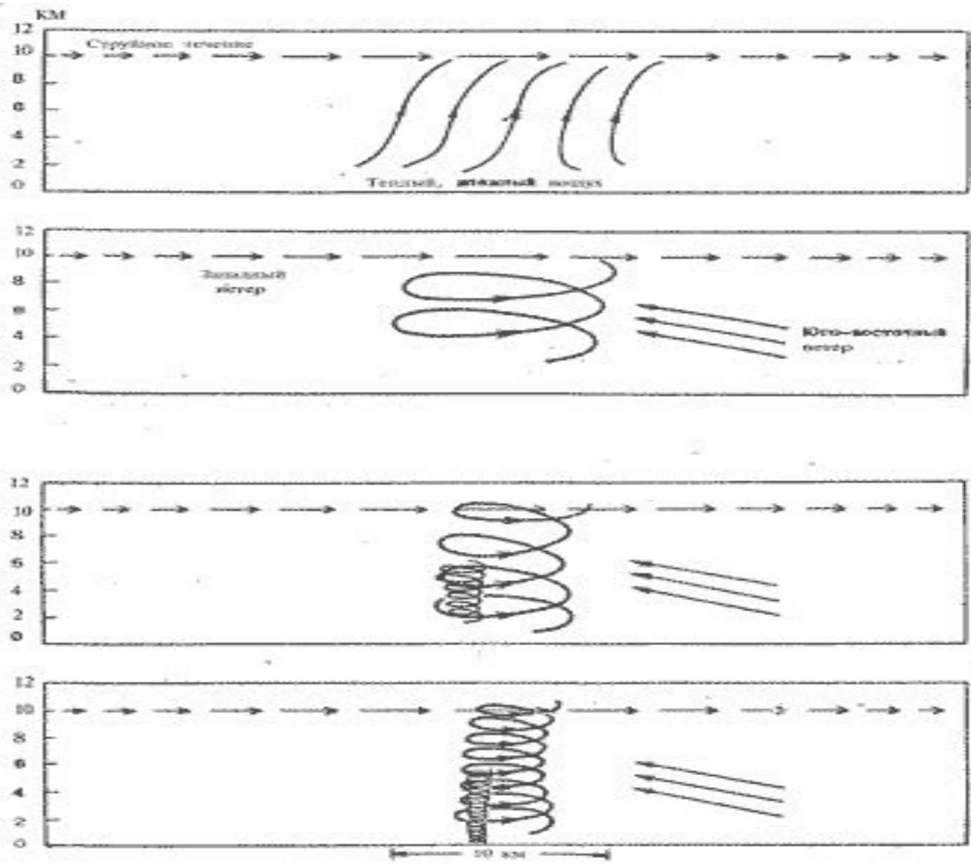
Рис. 1.2. Схема образования смерча по Д. Сноу [5]. Возмущенный поток воздуха при взаимодействии с ветром, имеющим большой вертикальный сдвиг скорости и направления, закручивается, формируя мелкомасштабный вихрь, в котором возникает смерч.
