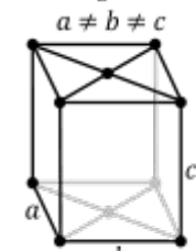
Базо-центрированная
