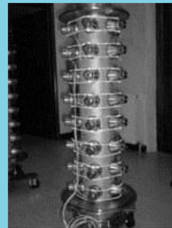
Аппарат для перекристаллизации при ультразвуковом воздействии
