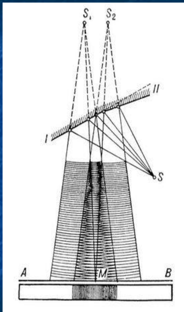
Зеркала Френеля
