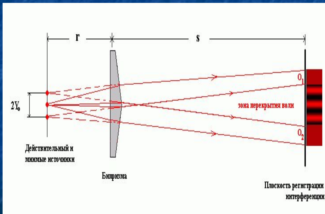
Бипризма Френеля
