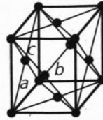
Гранецентрированная орторомбическая
