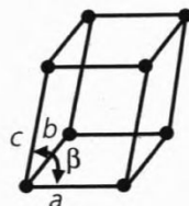
Простая моноклинная
