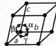
Триклинная
