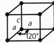
Гексагональная
