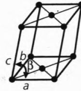
Базоцентрированная моноклинная
