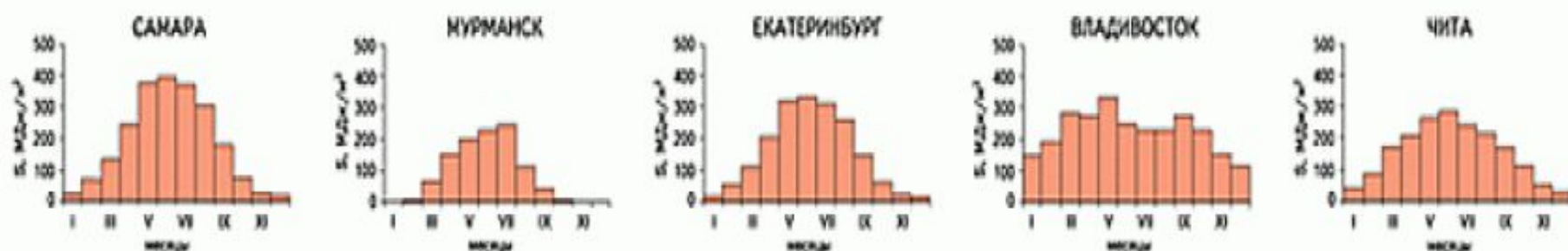
Годовой ход прямой солнечной радиации
