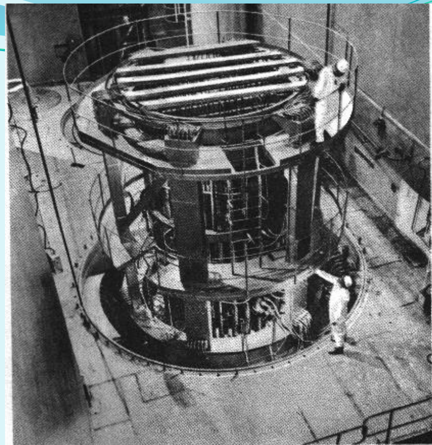
Рис. 56. Реактор Новovoroneжской АЭС (подготовка к работе).
