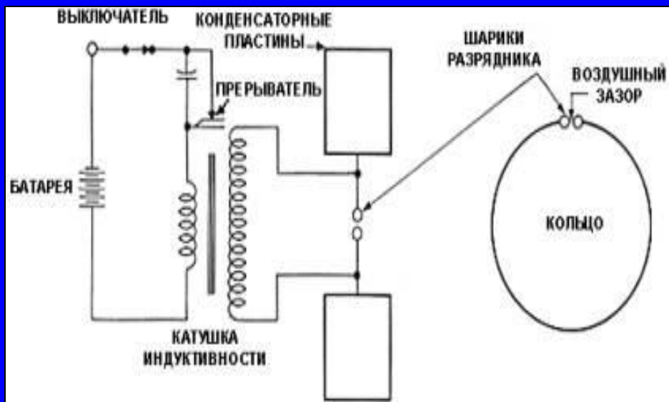
↑ вибратор (передатчик)
