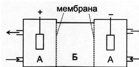
Схема электродиализатора
