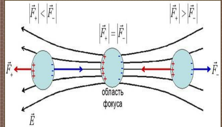
Оптический пинцет
