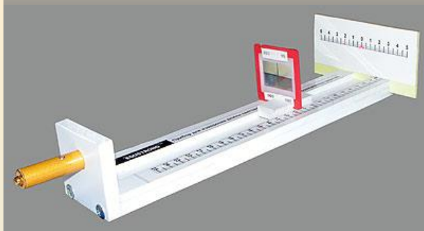
Определение длины световой волны с помощью дифракционной решетки
