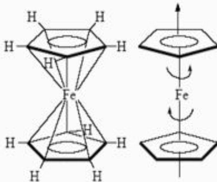
Ферроцен
