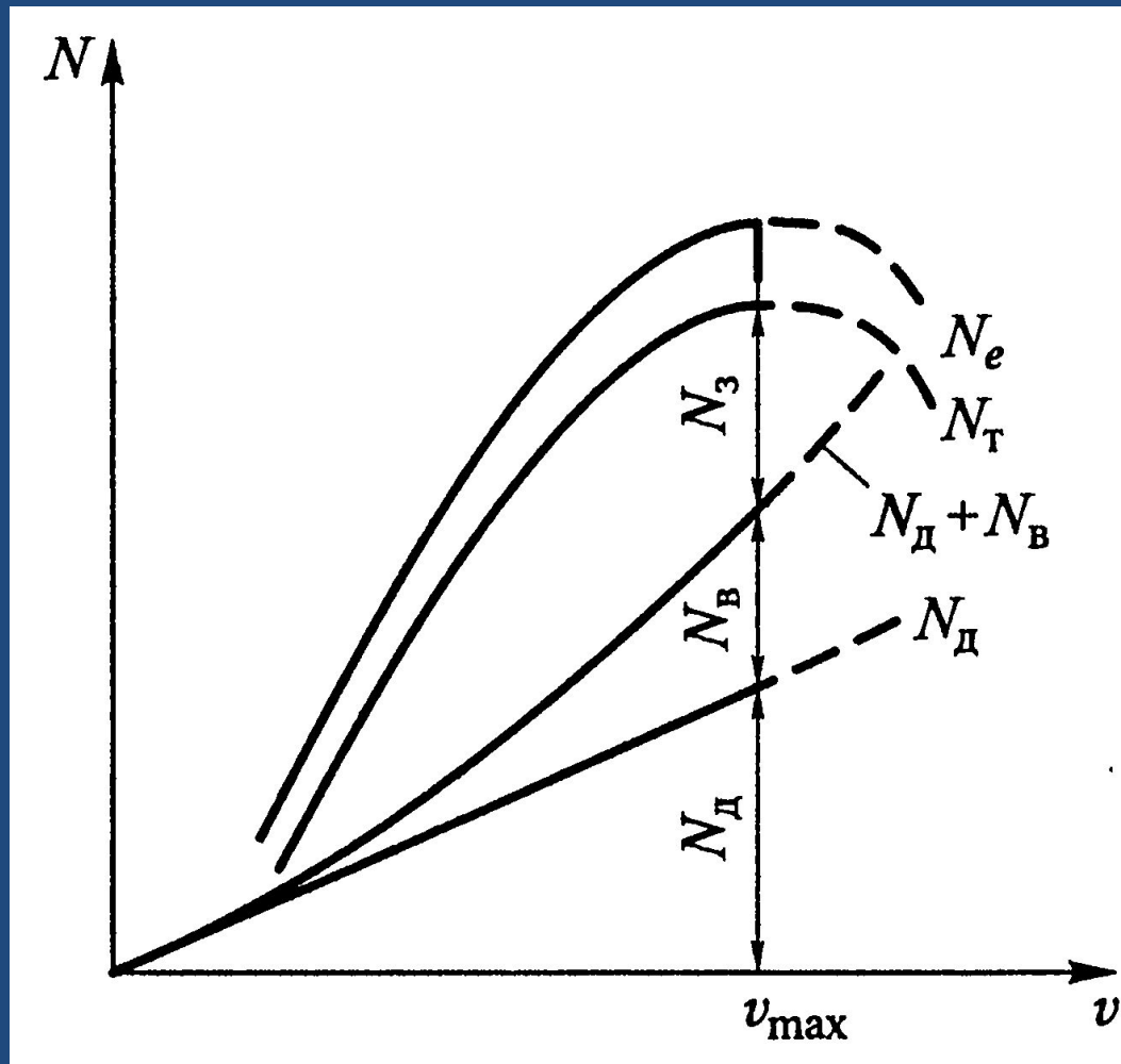
Рис. 3.27. График мощностного баланса автомобиля на высшей передаче
