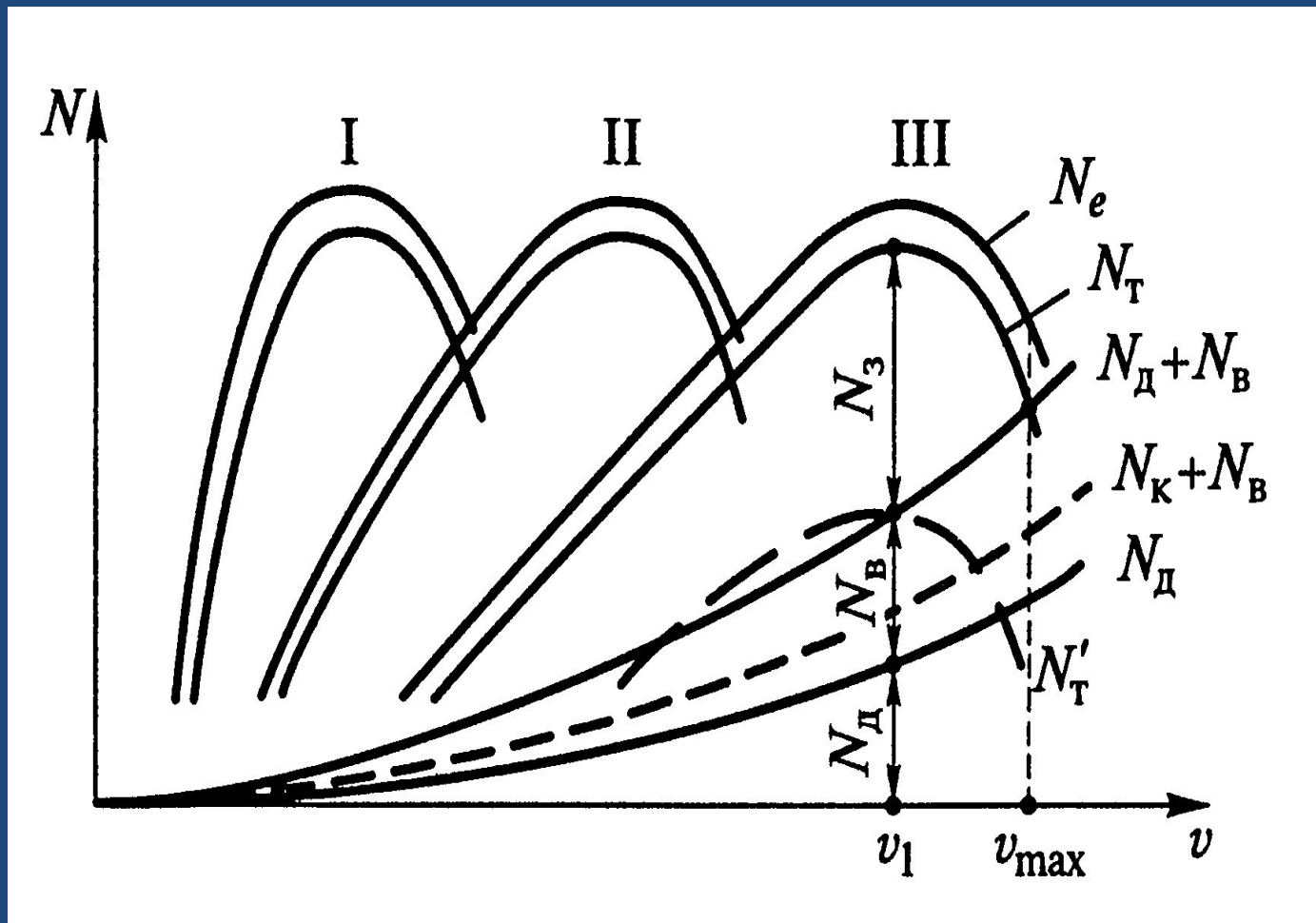
Рис. 3.26. График мощностного баланса автомобиля: N'_T - тяговая мощность на III передаче при уменьшенной подаче топлива; v , значение скорости автомобиля; I - III - передачи
