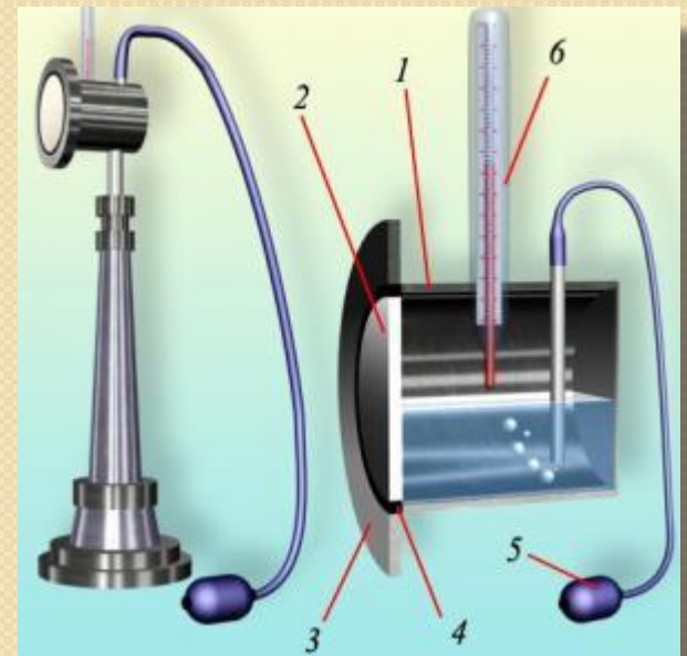
Конденсационный гигрометр
