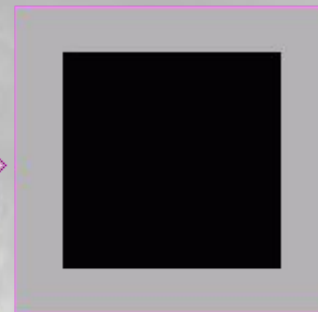
Нуль-мерный объект - континуальный вакуум
