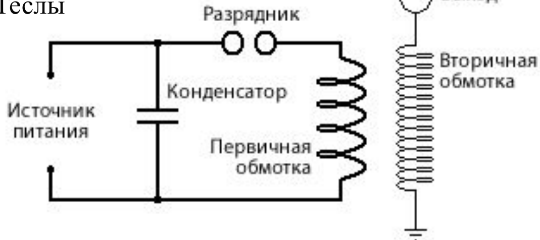
Трансформатор Теслы
