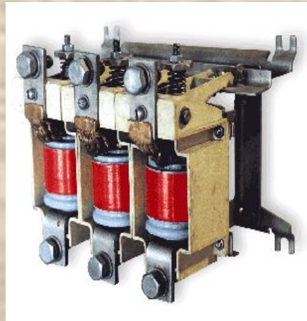
Контакторы вакуумные серии КТМ 15 на токи до 250 А
