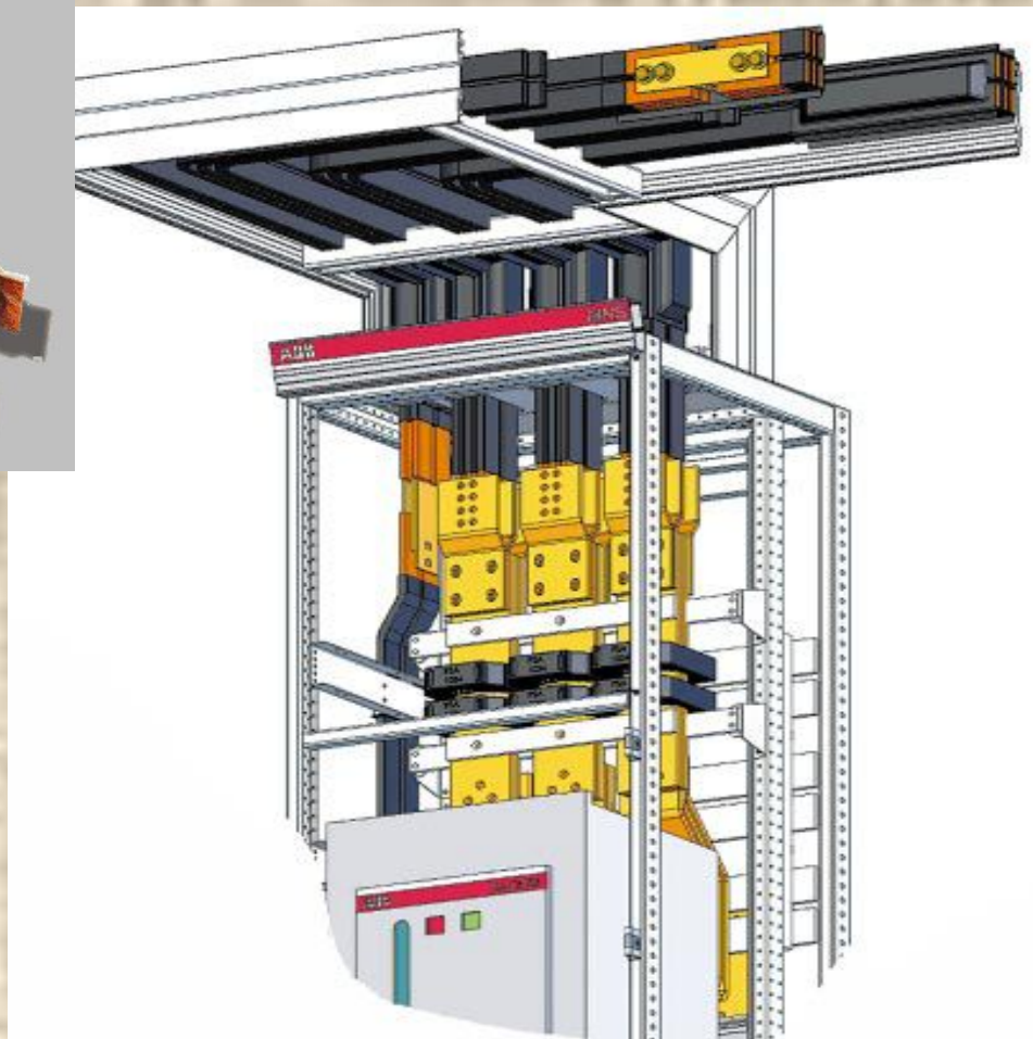
Секция магистрального шинопровода ШМА
