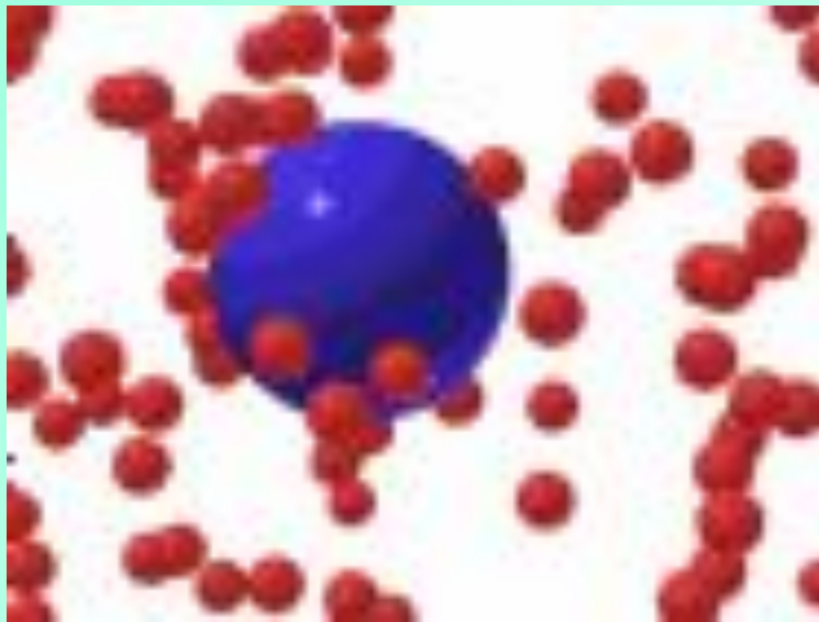
Броуновское движение
