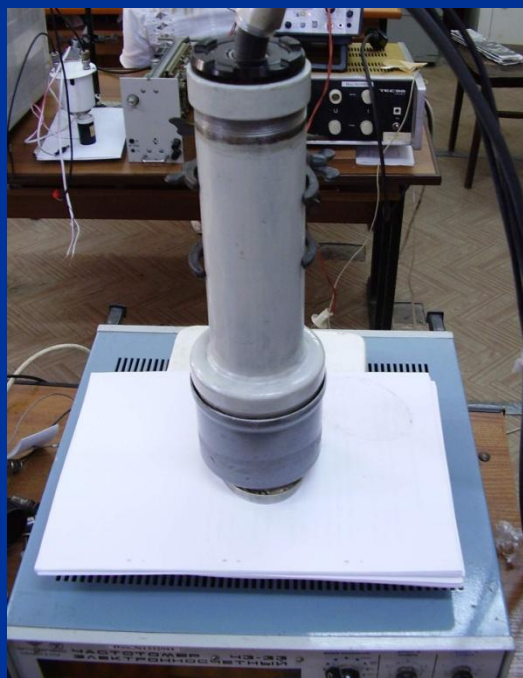
Рисунок 6 – Сцинтилляционный радиометр \alpha - частиц
