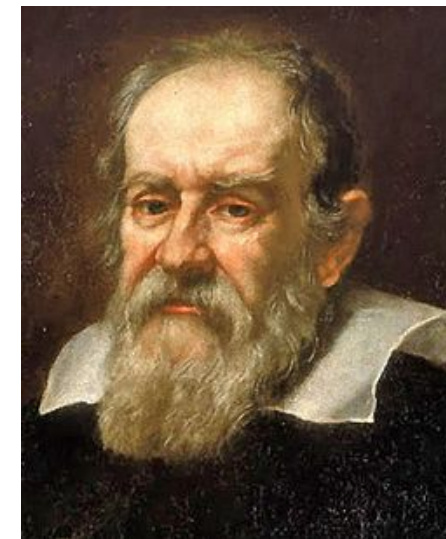
Галилео Галилей (1564- 1642)
