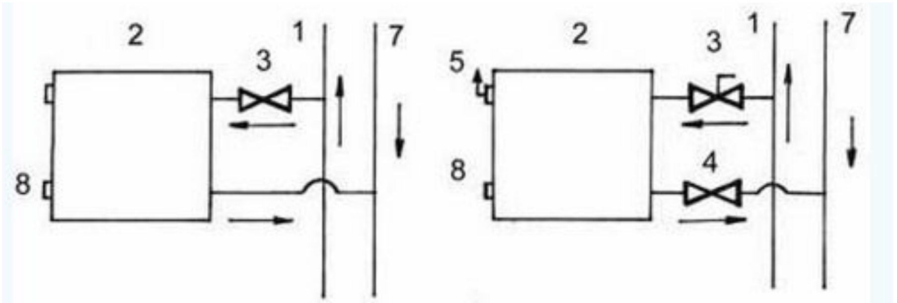
а – двухтрубная система стандартное подключение б - двухтрубная система рекомендуемое подключение
