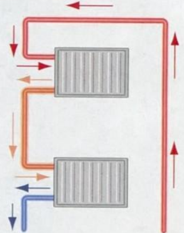
Однотрубная разводка
