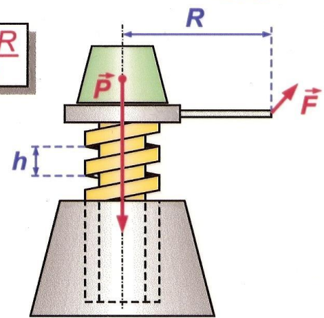
винтовой домкрат
