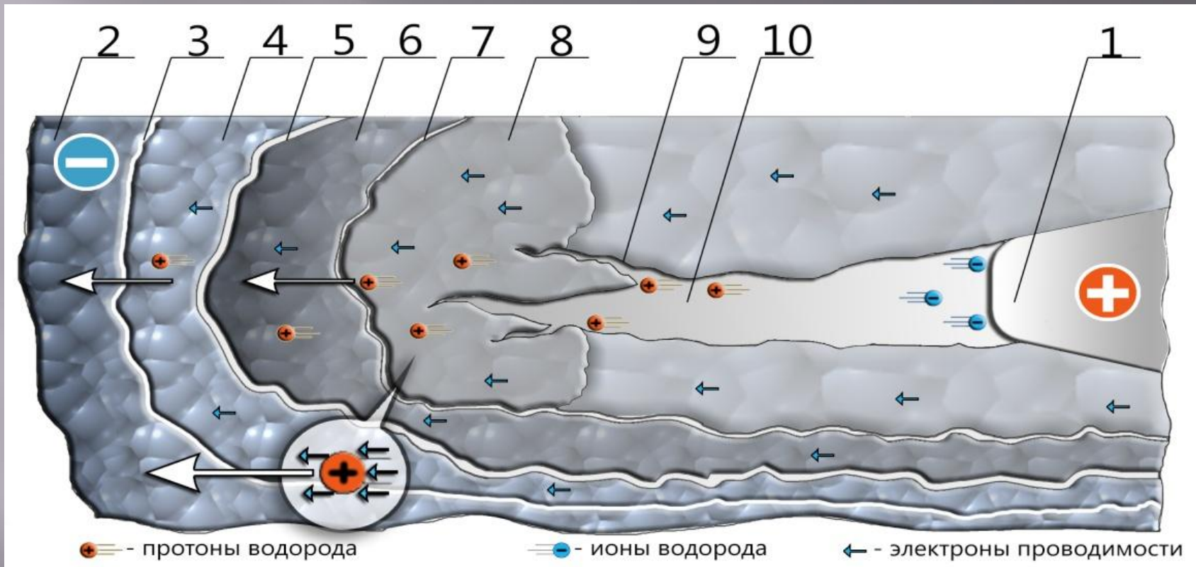
Рис.1. Схематическое изображение реакционной зоны. 1. Лезвие режущего инструмента; 2. Обрабатываемый металл; 3.Переходная область; 4. Область упругой деформации; 5. Область начального движения дислокаций; 6. Область пластической деформации; 7. Область докритического подрастания трещин; 8.Область разрушения. За критической стадией роста трещин; 9. Ювенильные полости трещин; 10. Магистральная трещина, заполненная водородной плазмой.
