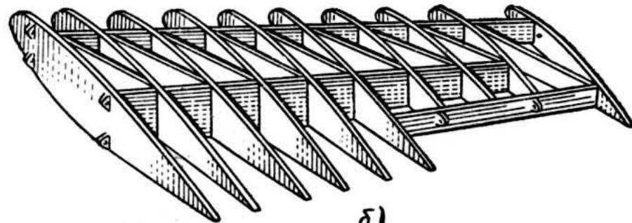
Отъемная часть крыла самолета а и ее монтажный эталон б
