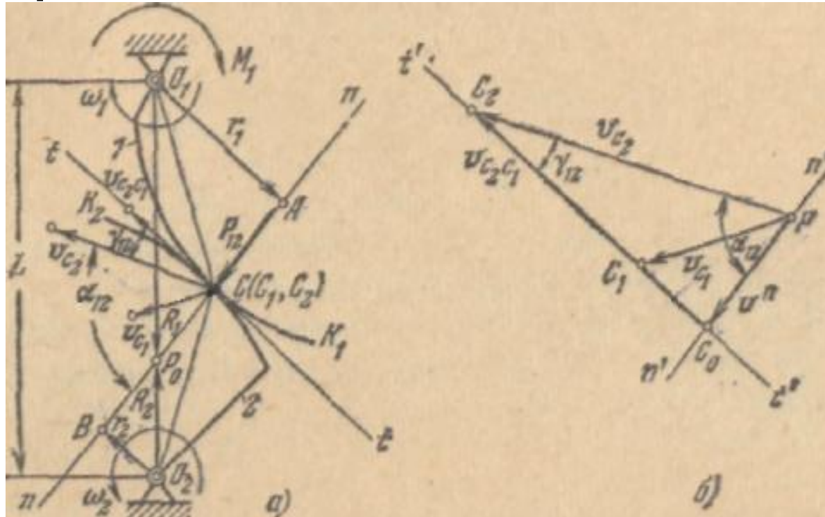
Рис 2 к определению форм профилей двух взаимноогibaемых кривых-, а) схема механизма с высшей парой; б) план скоростей.
