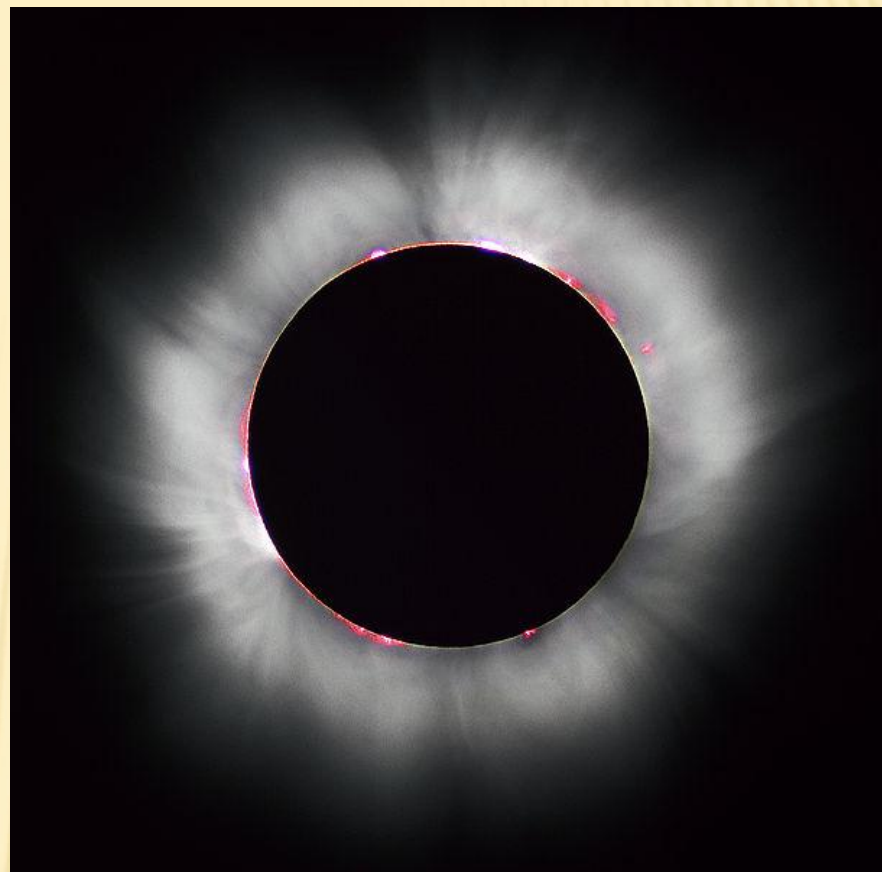
Солнечная корона во время солнечного затмения 1999 года
