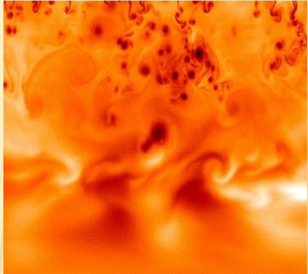
Зона конвекции Солнца
