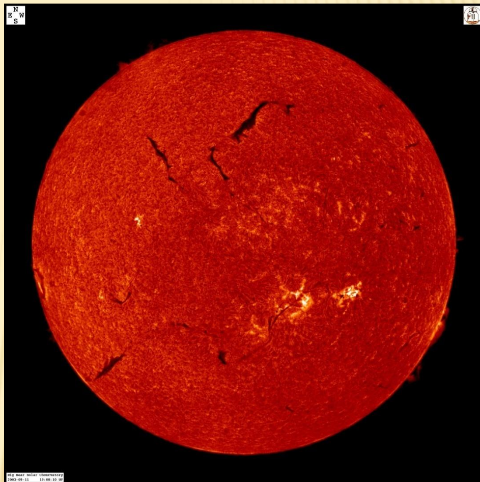
Хромосфера Солнца
