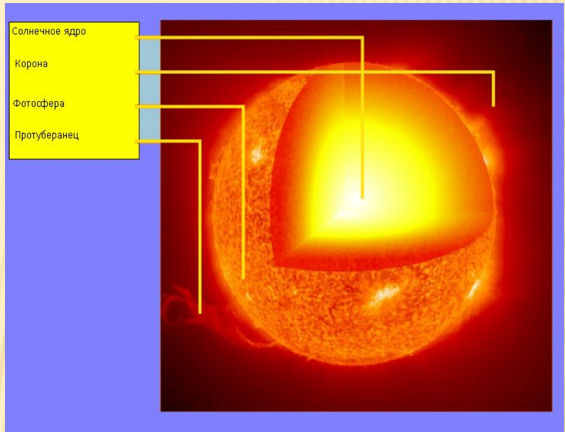
Схематичное строение Солнца
