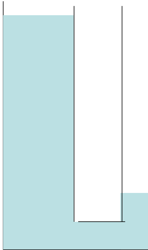
Вода-Ртуть
