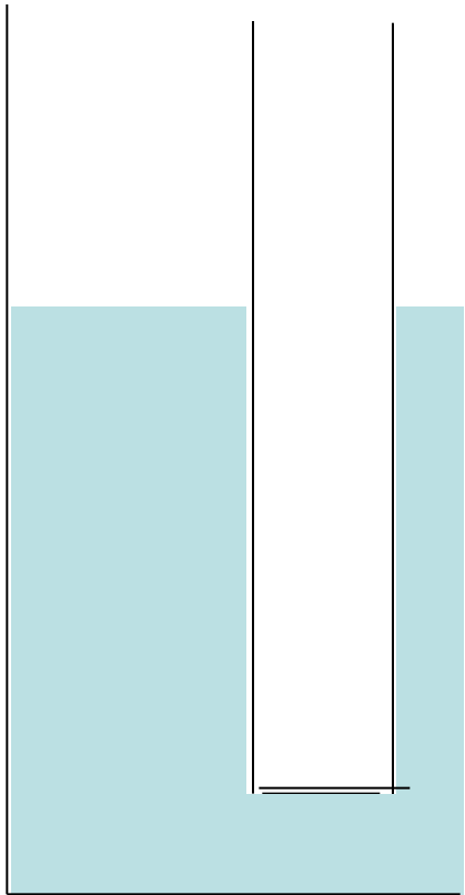
Вода-Вода
