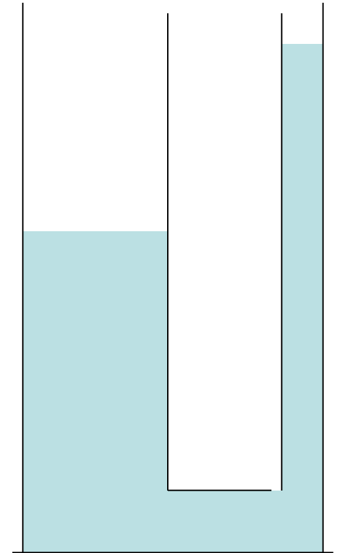
Вода-нефть
