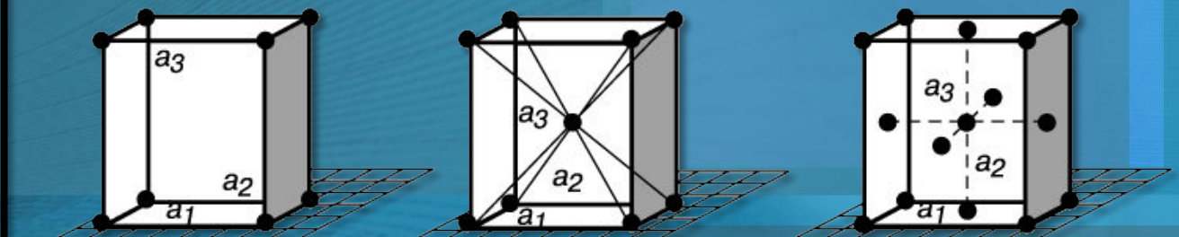
Кубическая
