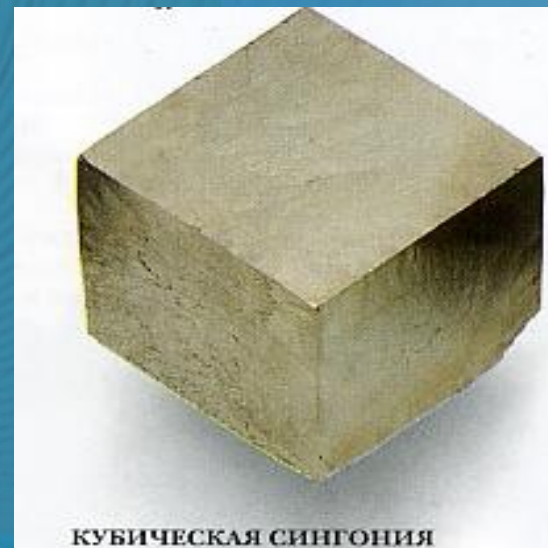
КУБИЧЕСКАЯ СИГНОНИЯ
