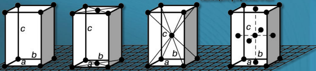
Орторомбическая
