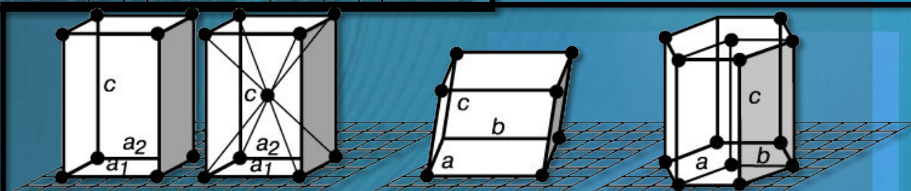
Тетрагональная
