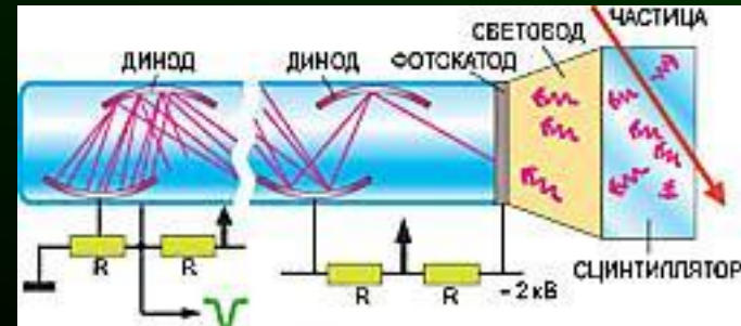
Сцинтилляционный счетчик
