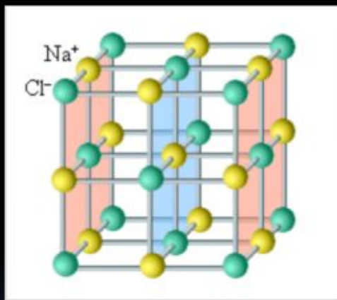
Кристаллическая решетка поваренной соли.
