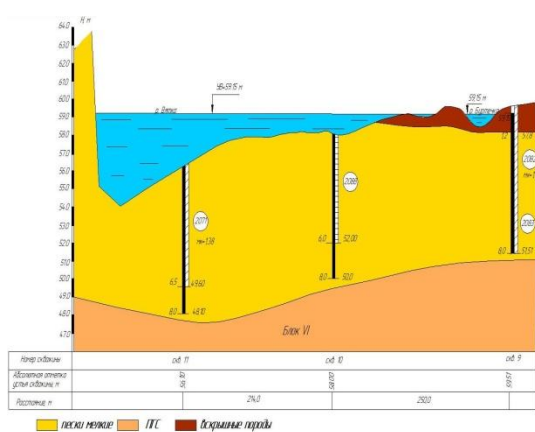
Геологический разрез XXII - XXII
