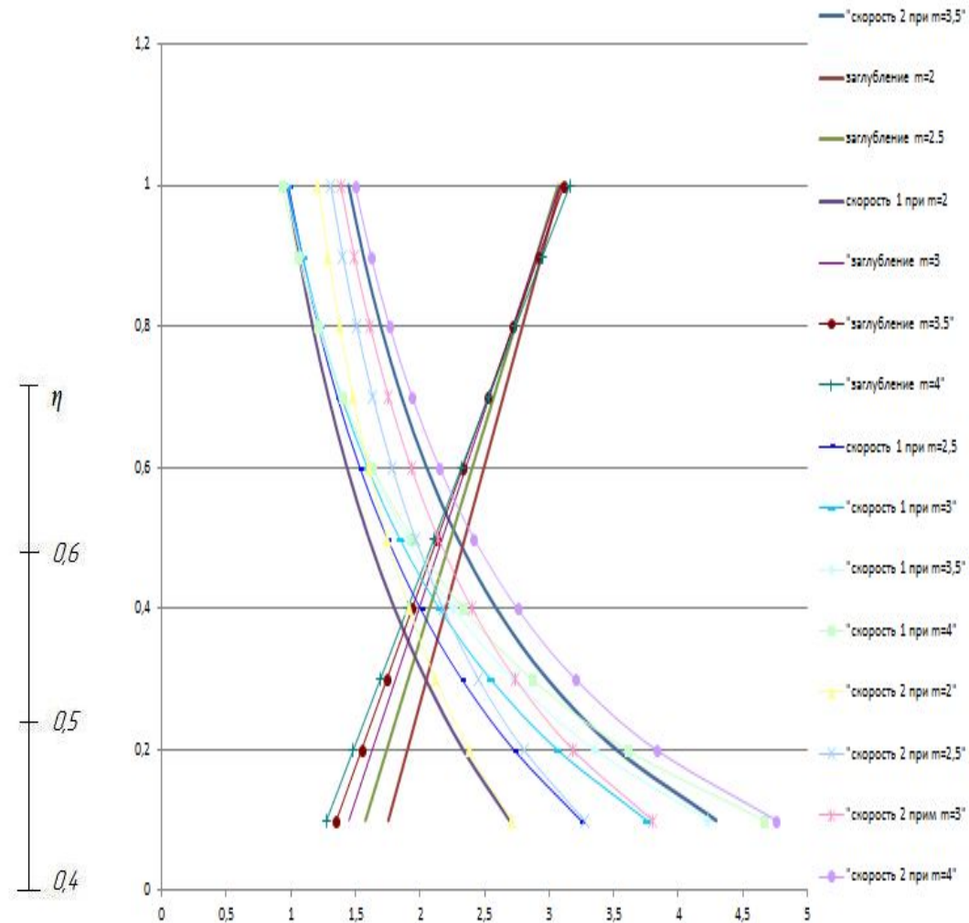
Технологическая карта работы земснаряда
